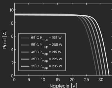
Charakterystyki temperaturowe
